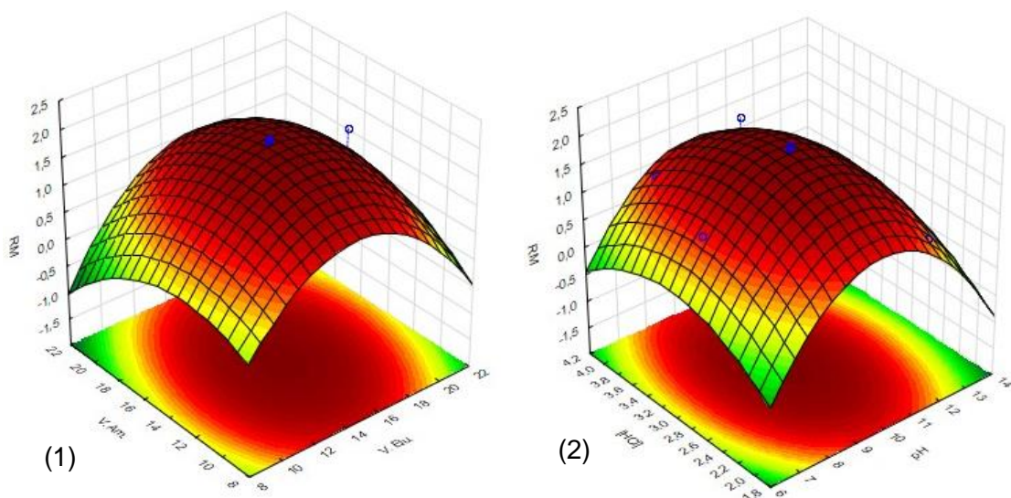
Figura 7: Superfícies de resposta, em 1 (RM x V. Am x V. Elu); em 2 (RM x [HCl] x pH)
