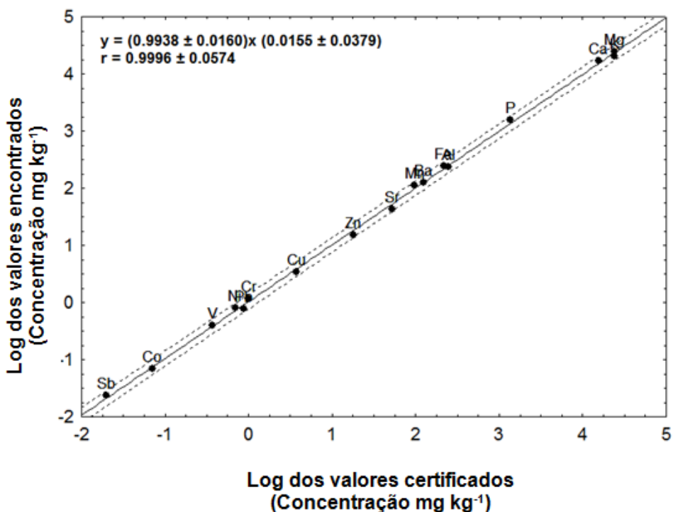
Figura 2.5. Gráfico de regressão linear para análise do CRM de Folha de pessegueiro (NIST 1547): Al, Ba, Ca, Co, Cr, Cu, Fe, K, Mg, Mn, Ni, P, Pb, Sb, Sr, V e Zn.
