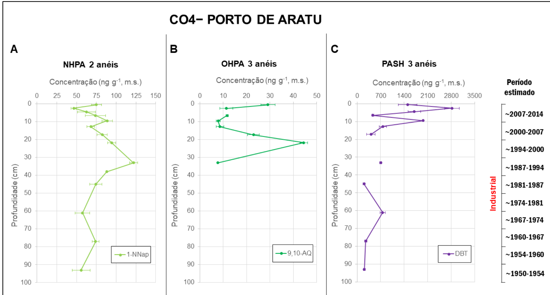
Figura 14– Perfis do 1-nitronaftaleno (1-NNap), 9,10-antraquinona (9,10-AQ) e dibenzotiofeno (DBT) nos sedimentos do testemunho CO4 coletado na área do Porto de Aratu. No lado direito encontra-se a escala temporal estimada (ano), mostrando o período industrial (> 1940) na BTS.
