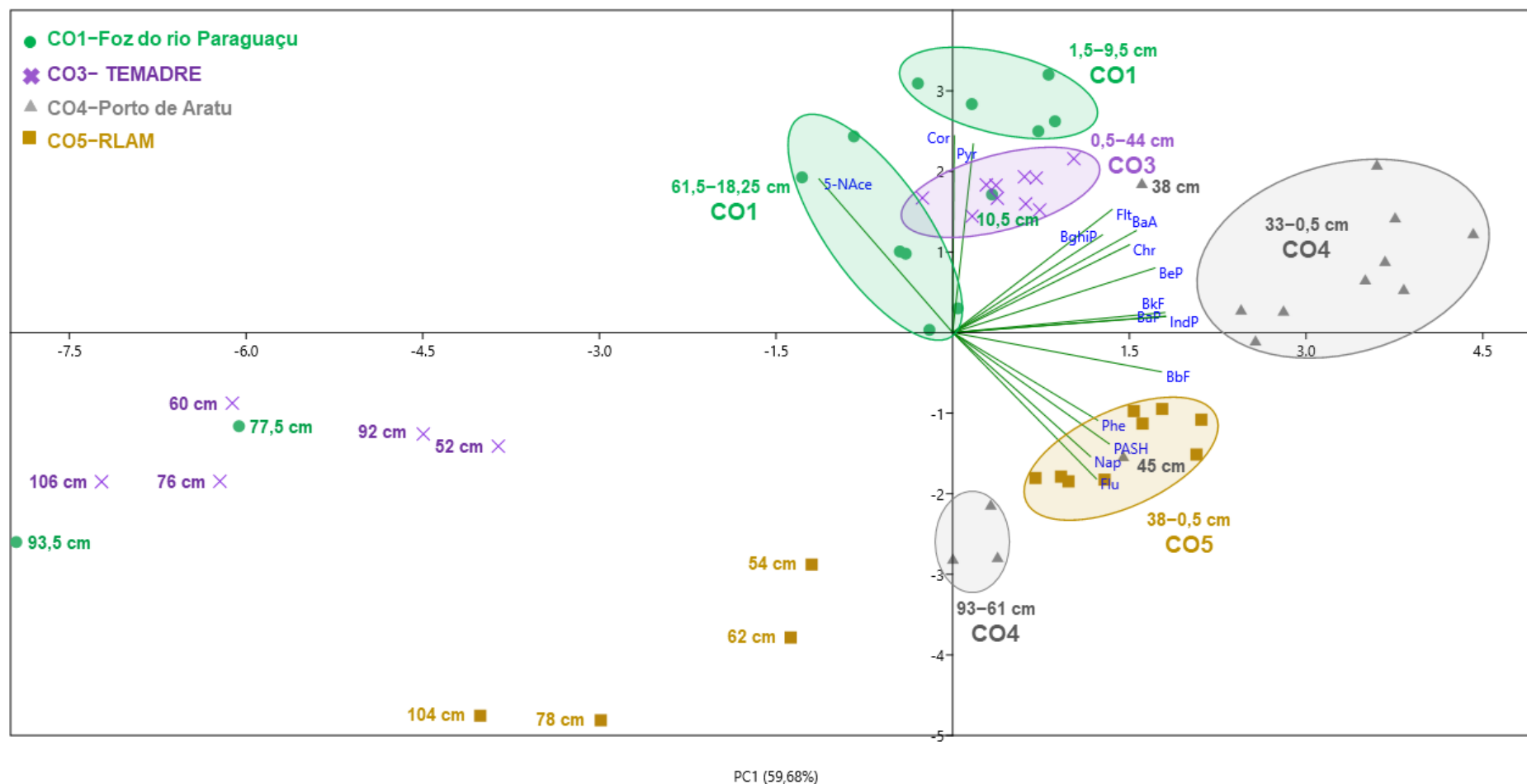
Figura 17 – Pesos dos componentes principais do PCA com base nos dados de HPA e derivados normalizados e padronizados dos testemunhos CO1–Foz do rio Paraguaçu (●), TEMADRE–CO3 (X), Porto de Aratu–CO4 (▲) e Refinaria RLAM–CO5 (■) da BTS. Como auxílio visual foram usadas elipses para agrupar algumas amostras em cada testemunho. O Biplot são projeções dos eixos originais (variáveis)
